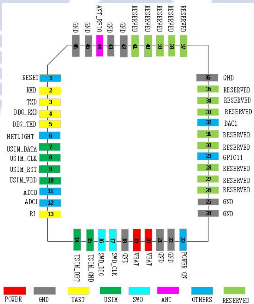
图1 管脚示意图
