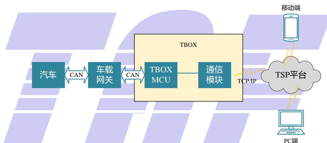
图1 TBOX结构与逻辑示意图
